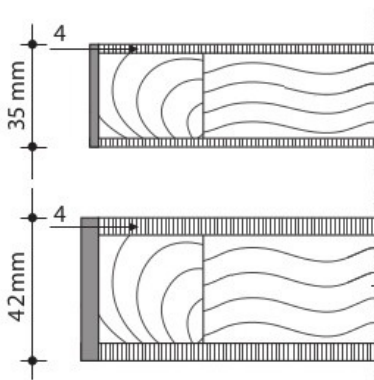
DETALHE EM PLANTA
